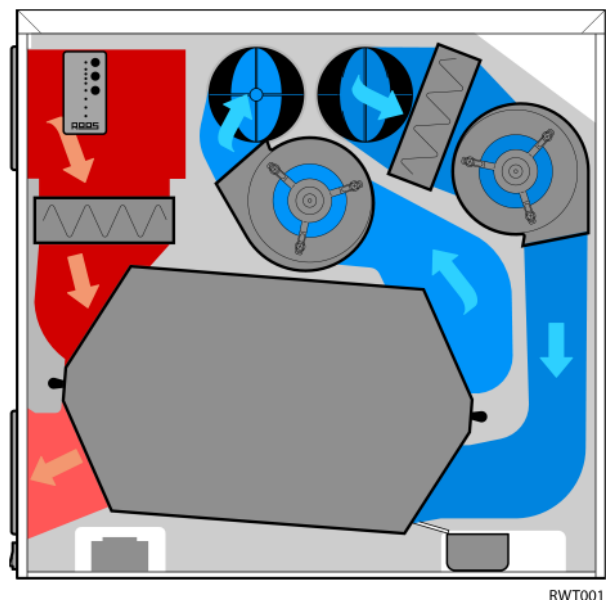
Abbildung 1: Funktionsschema
